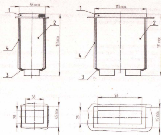
Рисунок А.1 - Устройство табло.
